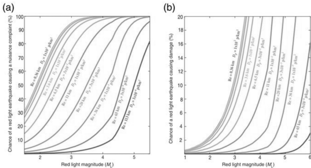
图3 各种 TLP 模拟场景下的风险曲线
