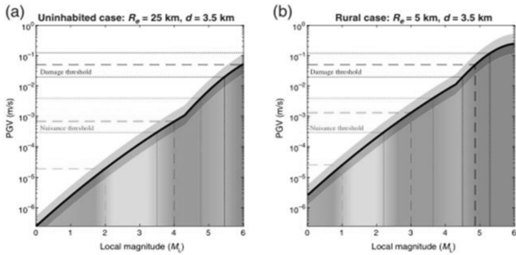
图2 PGV 与 ML 的比例关系
