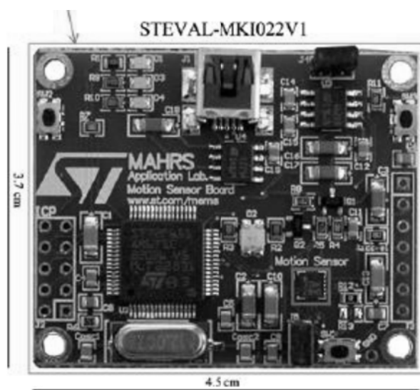
图 1 STEVAL-MKI022V1 套件，其上搭载了 LIS331DLH 运动传感器(红色方框)
