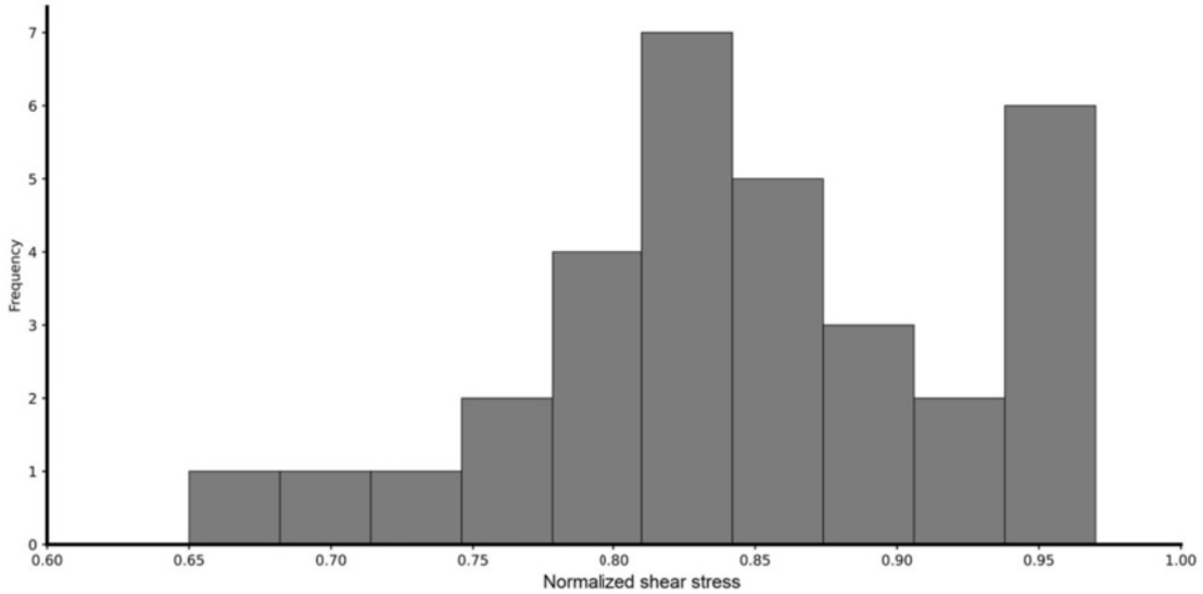
图 4 8 级以上地震发生前的标准化剪切应力值的分布
