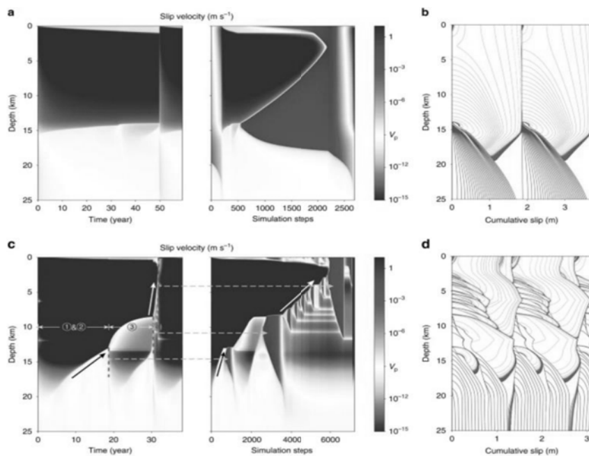
图 1 滑移速率和滑移行为的变化
